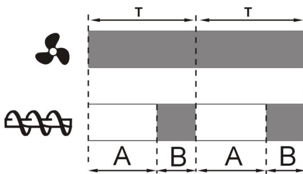
Obr. č.6 Pracovní cykly ventilátoru a podavače v režimu PROVOZ
