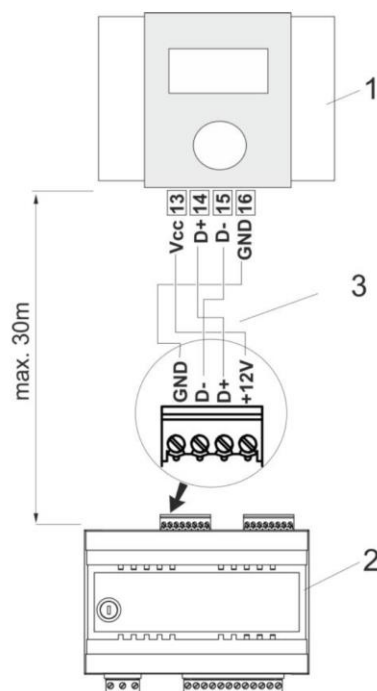
Obr. č.15 4-žilové zapojení pokojového panelu
