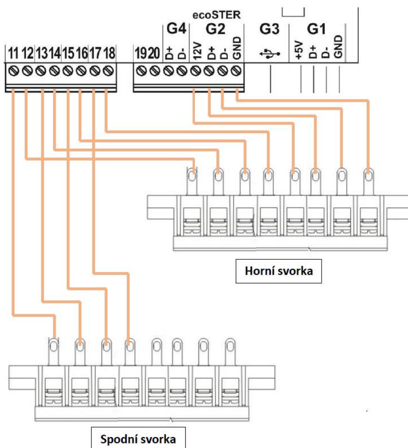
Obr. č.12 Schéma zapojení čidel
