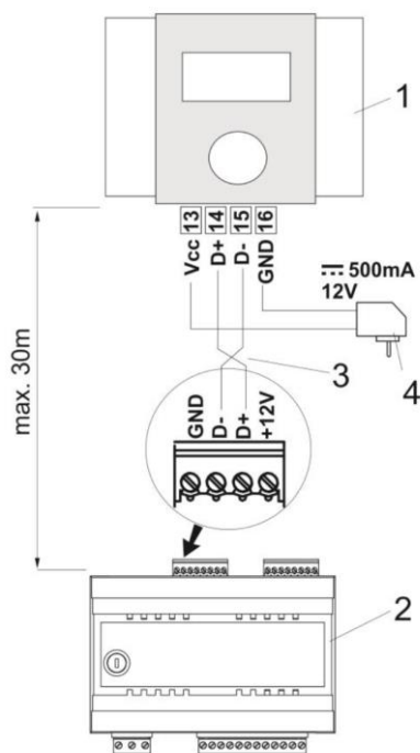
Obr. č.16 2-žilové zapojení pokojového panelu
