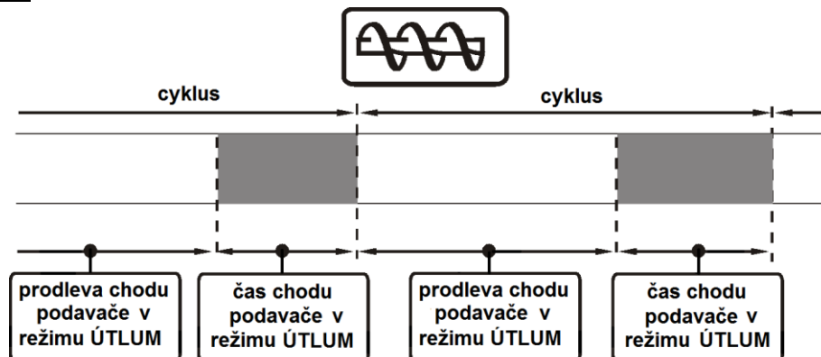
Obr. č.8 Pracovní cykly podavače paliva v režimu ÚTLUM
