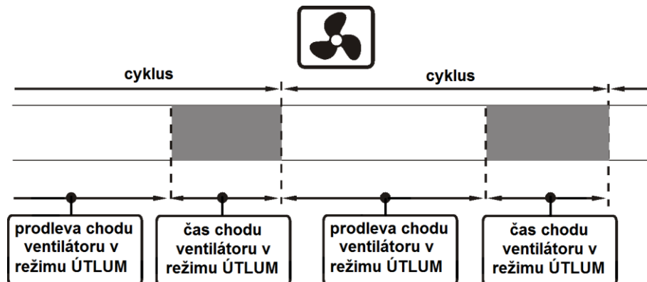
Obr. č.7 Pracovní cykly ventilátoru v režimu ÚTLUM
