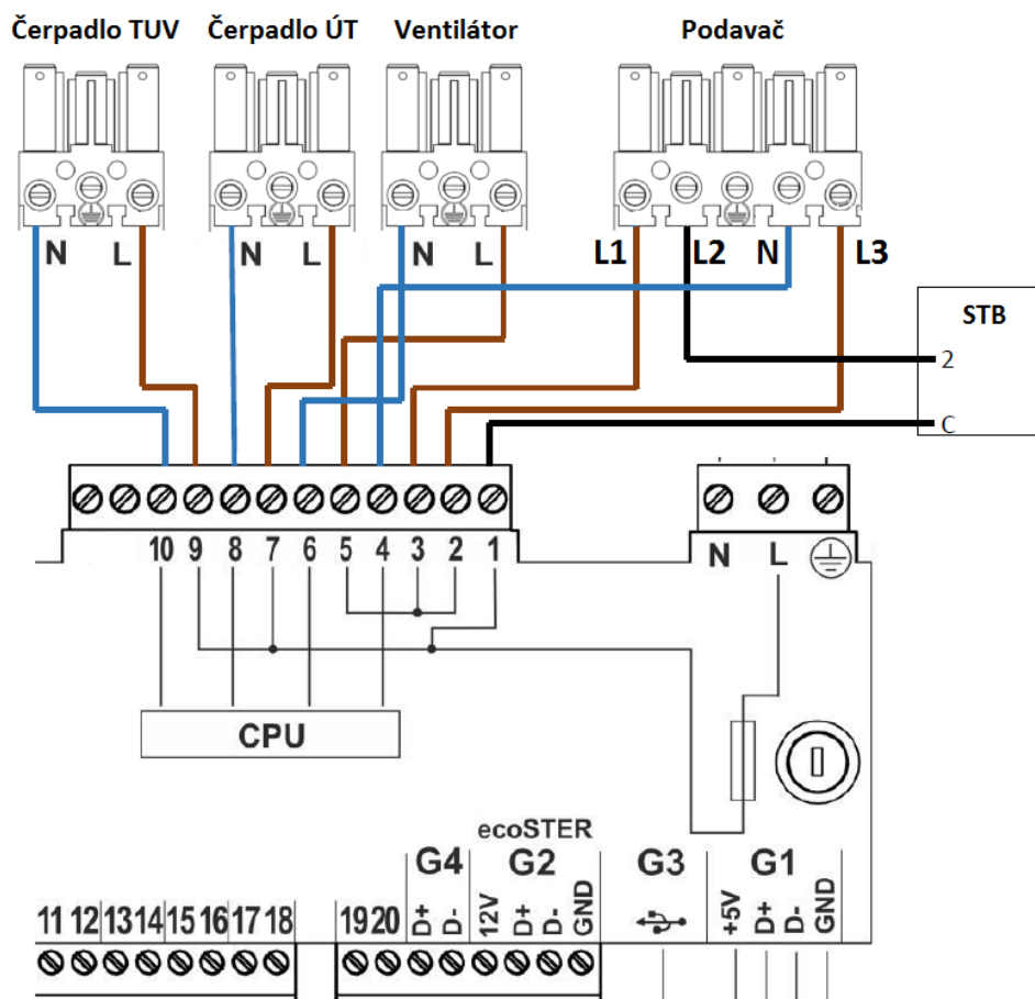
Obr. č.13 Schéma zapojení konektorů
