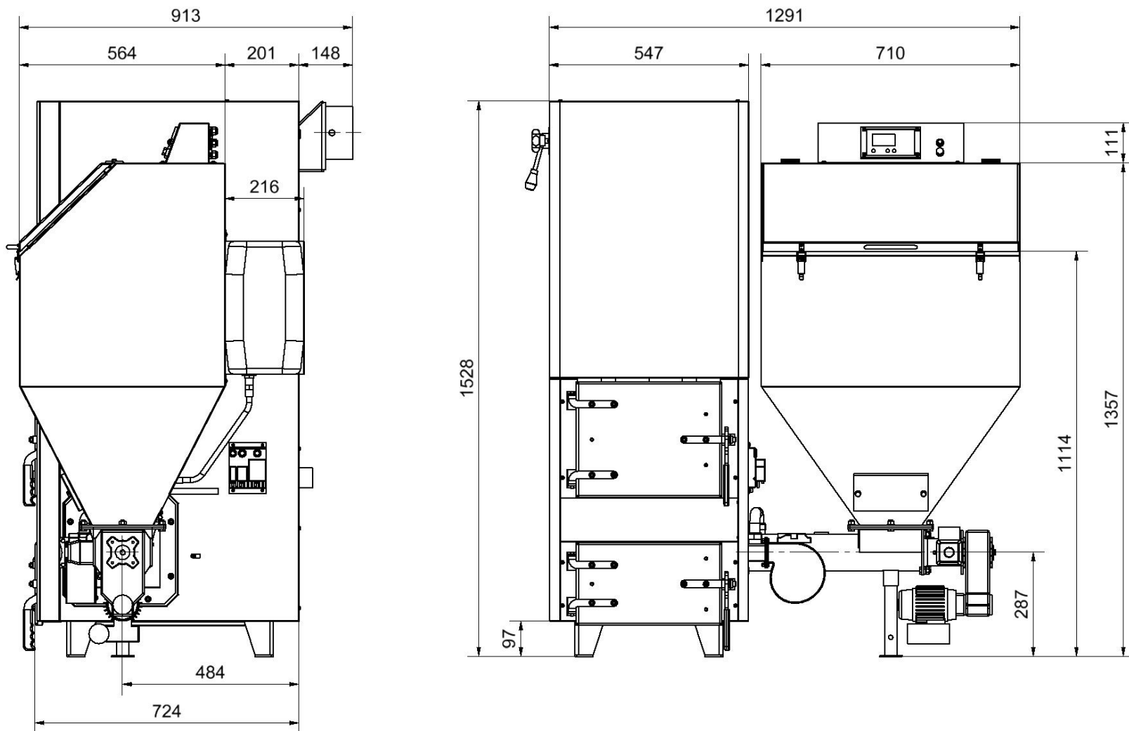
Obr. č. 3 Základní rozměry kotle CosmoTHERM U25 se zásobníkem 280l
