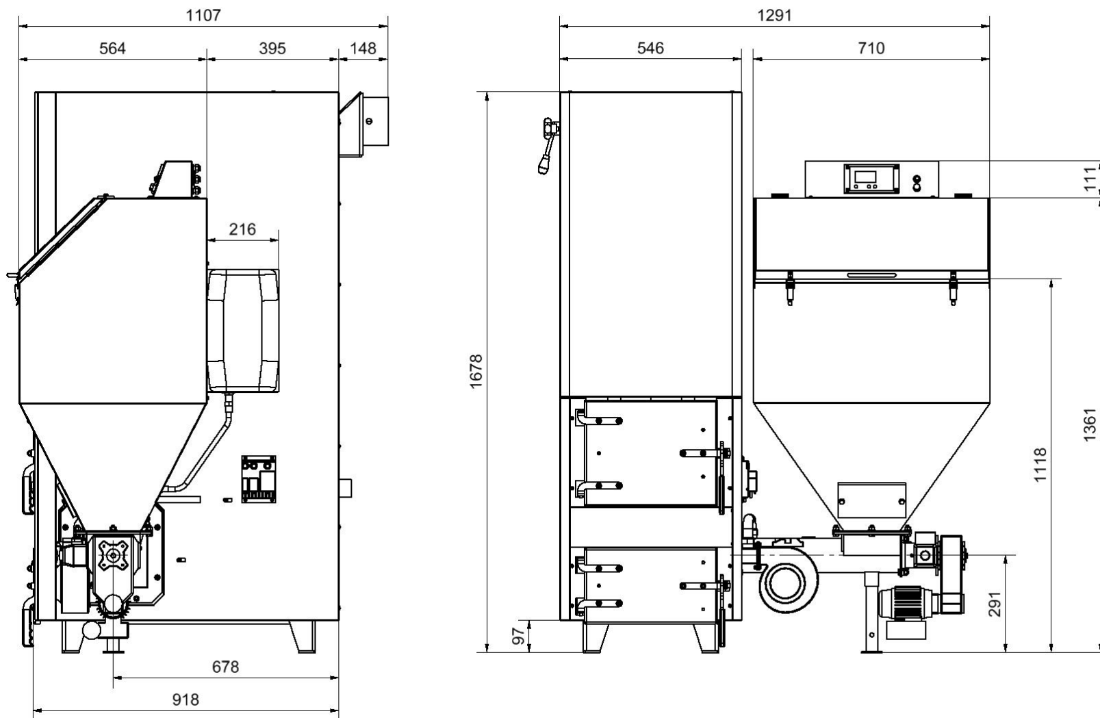
Obr. č. 5 Základní rozměry kotle CosmoTHERM U35 se zásobníkem 280l
