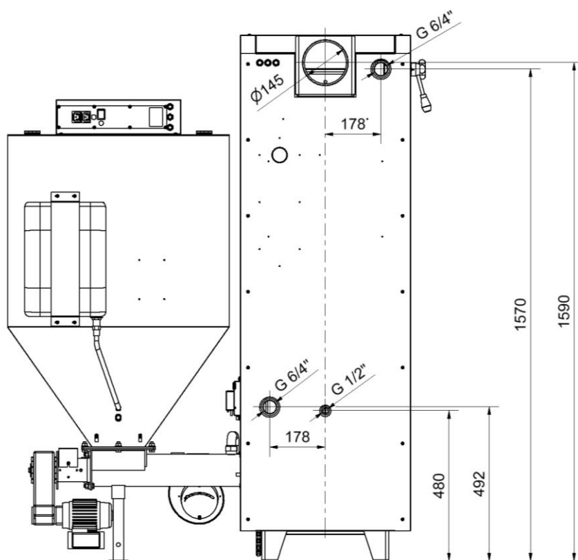
Obr. č. 10 Připojovací rozměry kotle CosmoTHERM U35
