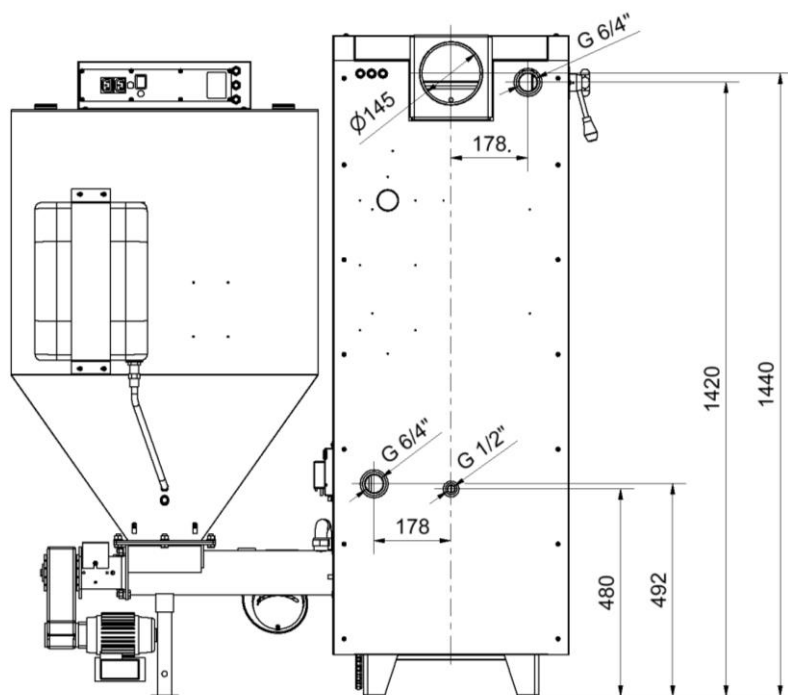
Obr. č. 9 Připojovací rozměry kotle CosmoTHERM U25
