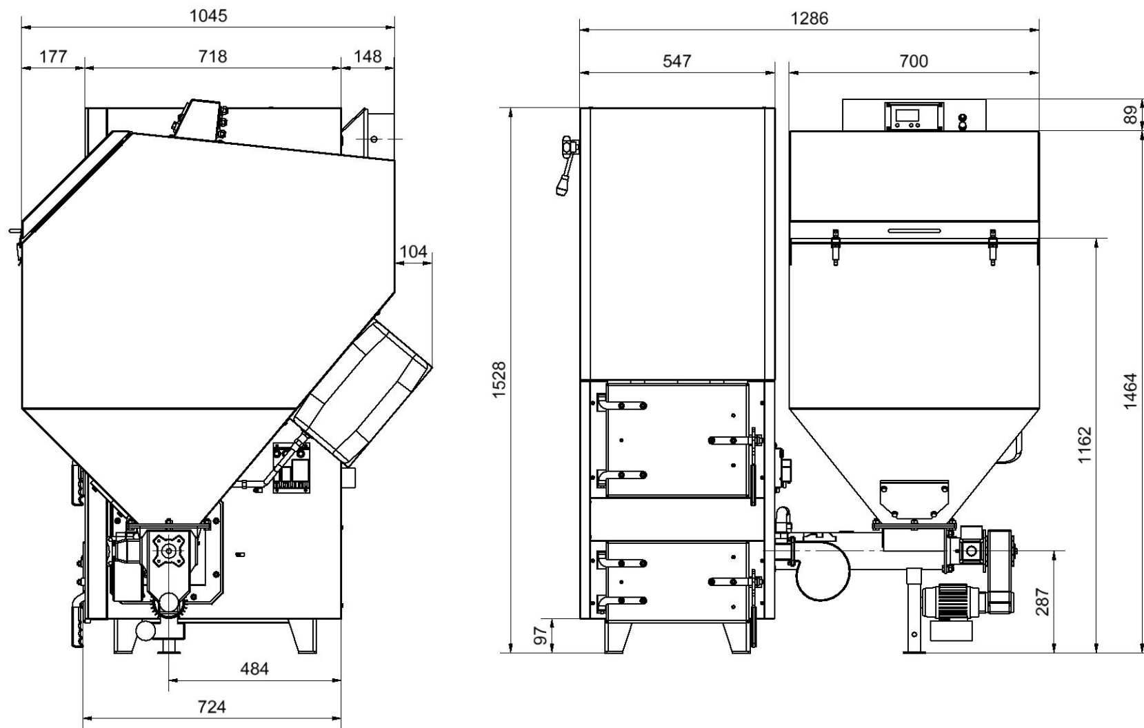
Obr. č. 6 Základní rozměry kotle CosmoTHERM U35 se zásobníkem 540I
