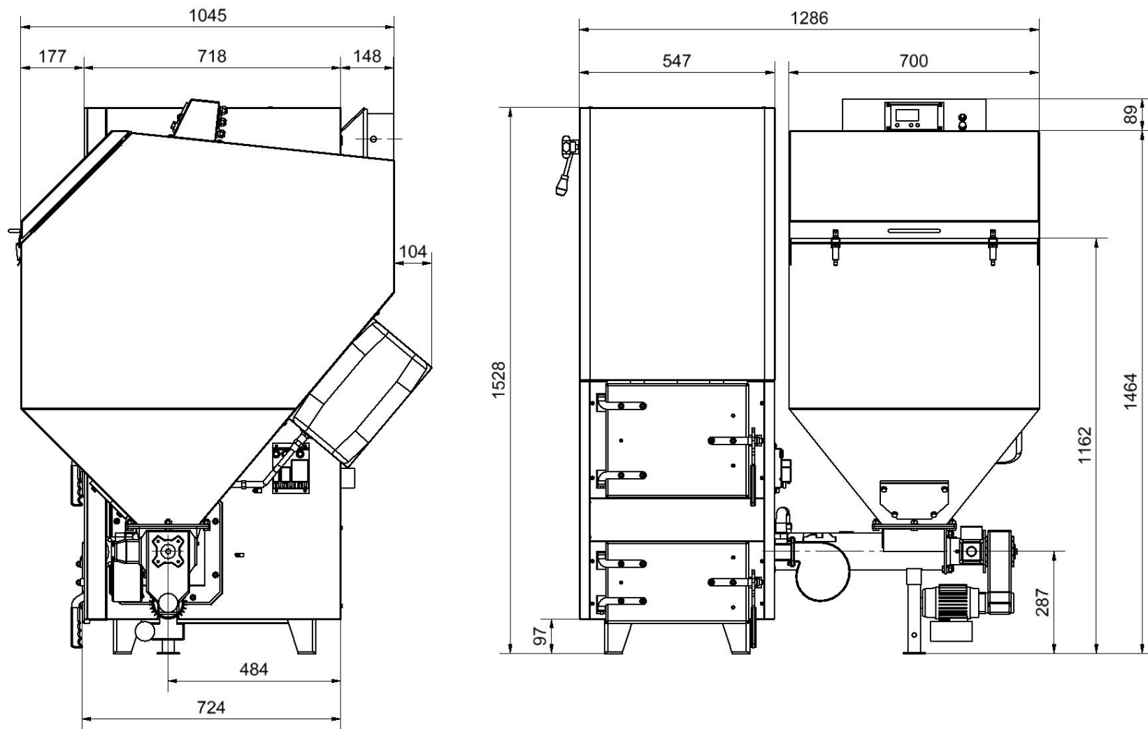
Obr. č. 4 Základní rozměry kotle CosmoTHERM U25 se zásobníkem 540I
