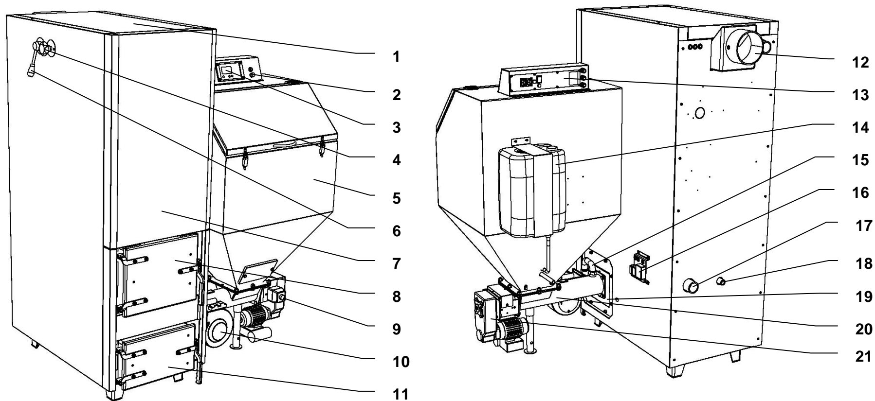
Obr. č. 2 Čelní a zadní pohled kotle CosmoTHERM U35
