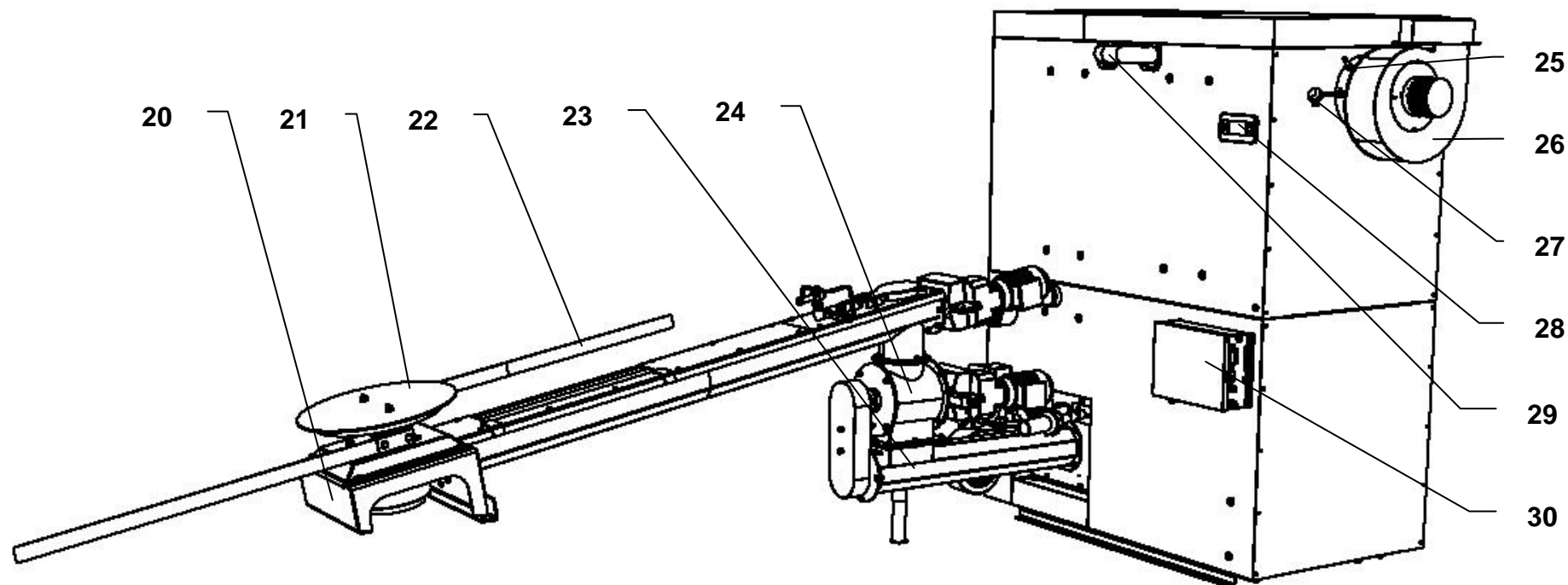
Obr. č. 2 Zadní pohled kotle BENEKOV S100
