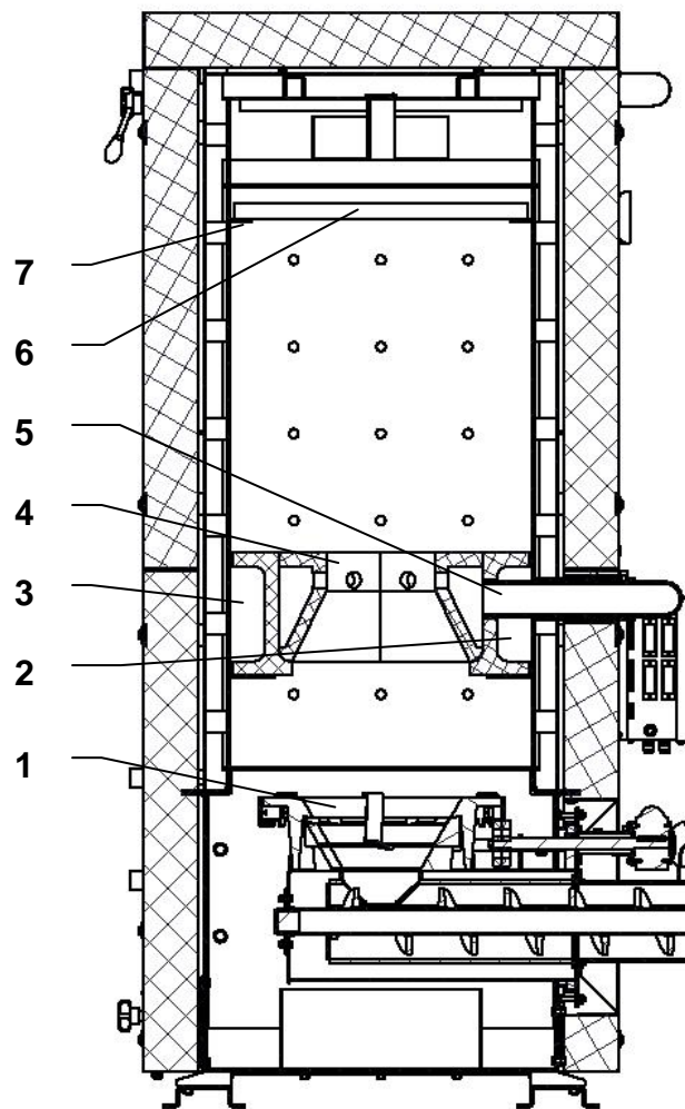
Obr. č. 9 Řez spalovací komorou kotle
