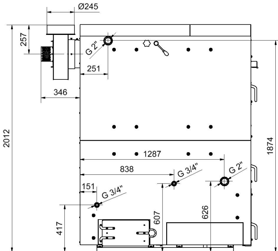
Obr. č. 8 Připojovací rozměry kotle BENEKOV S100
