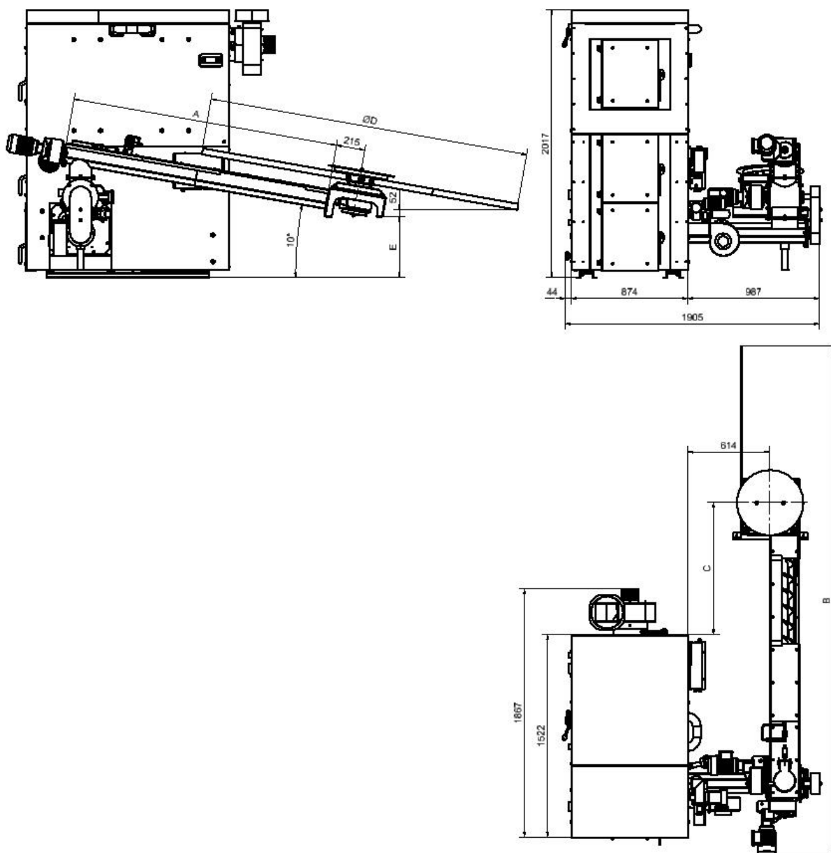
Obr. č. 5 Základní rozměry kotle BENEKOV S100 se zadním uspořádáním podávání z bunkru
