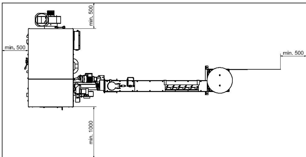
Obr. č. 6 Umístění kotle v kotelně
