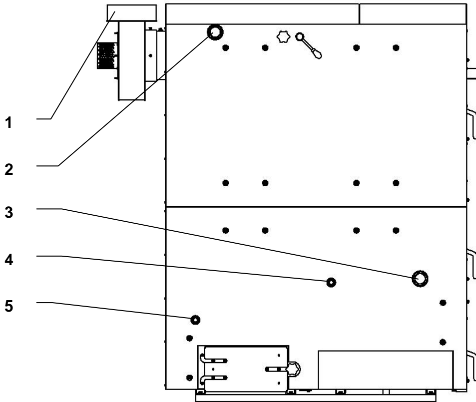
Obr. č. 7 Vstupy a výstupy kotle BENEKOV S100
