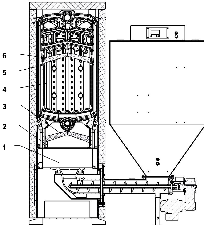
Obr. č. 7 Řez kotlem
