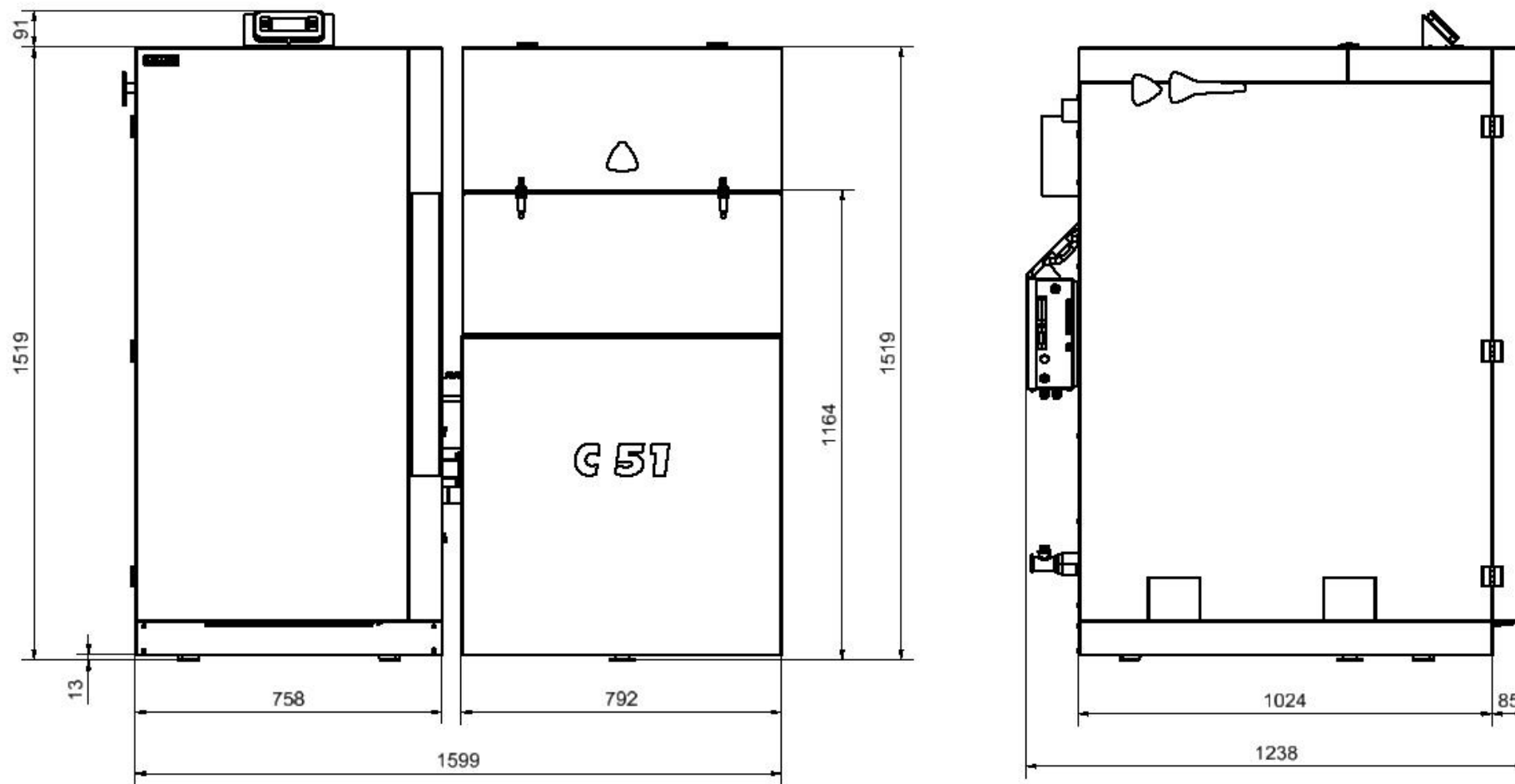
Obr. č. 6 Základní rozměry kotle BENEKOV C51
