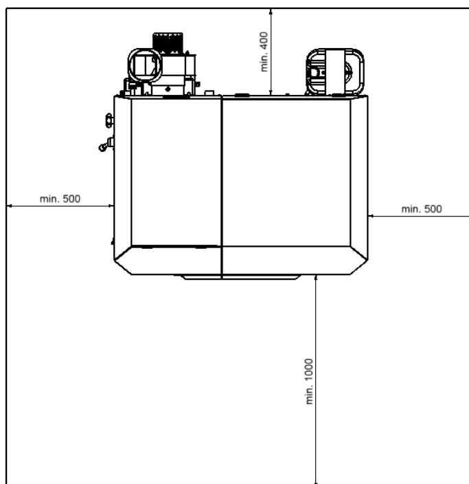
Obr. č. 5 Umístění kotle v kotelně
