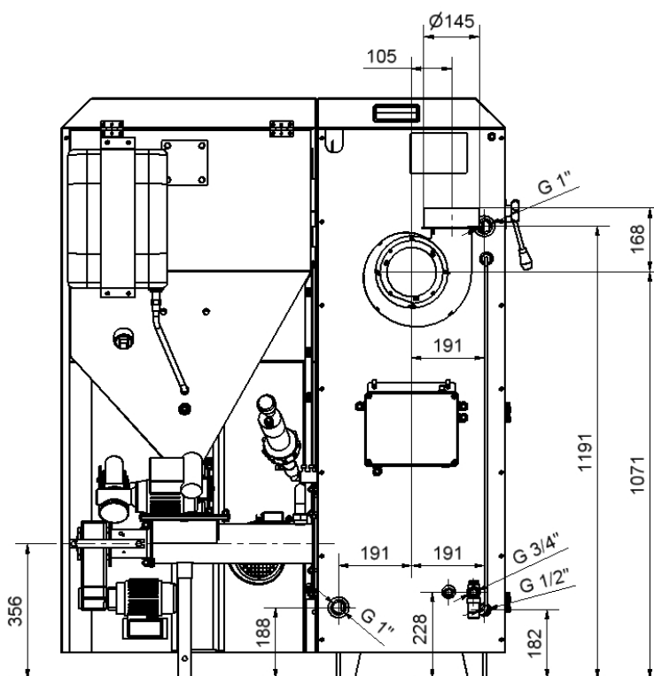
Obr. č. 7 Připojovací rozměry kotle CosmoTHERM G25
