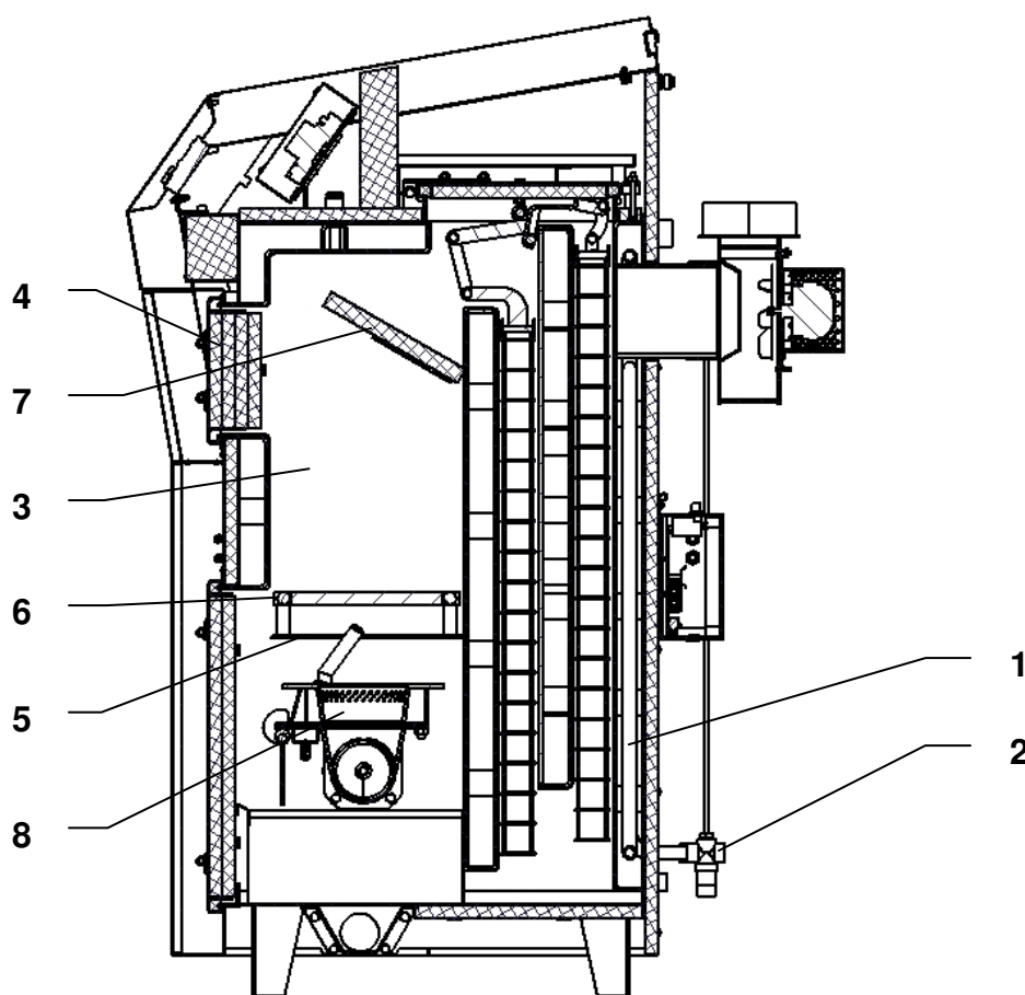
Obr. č. 9 Umístění přídavného roštu do kotle
