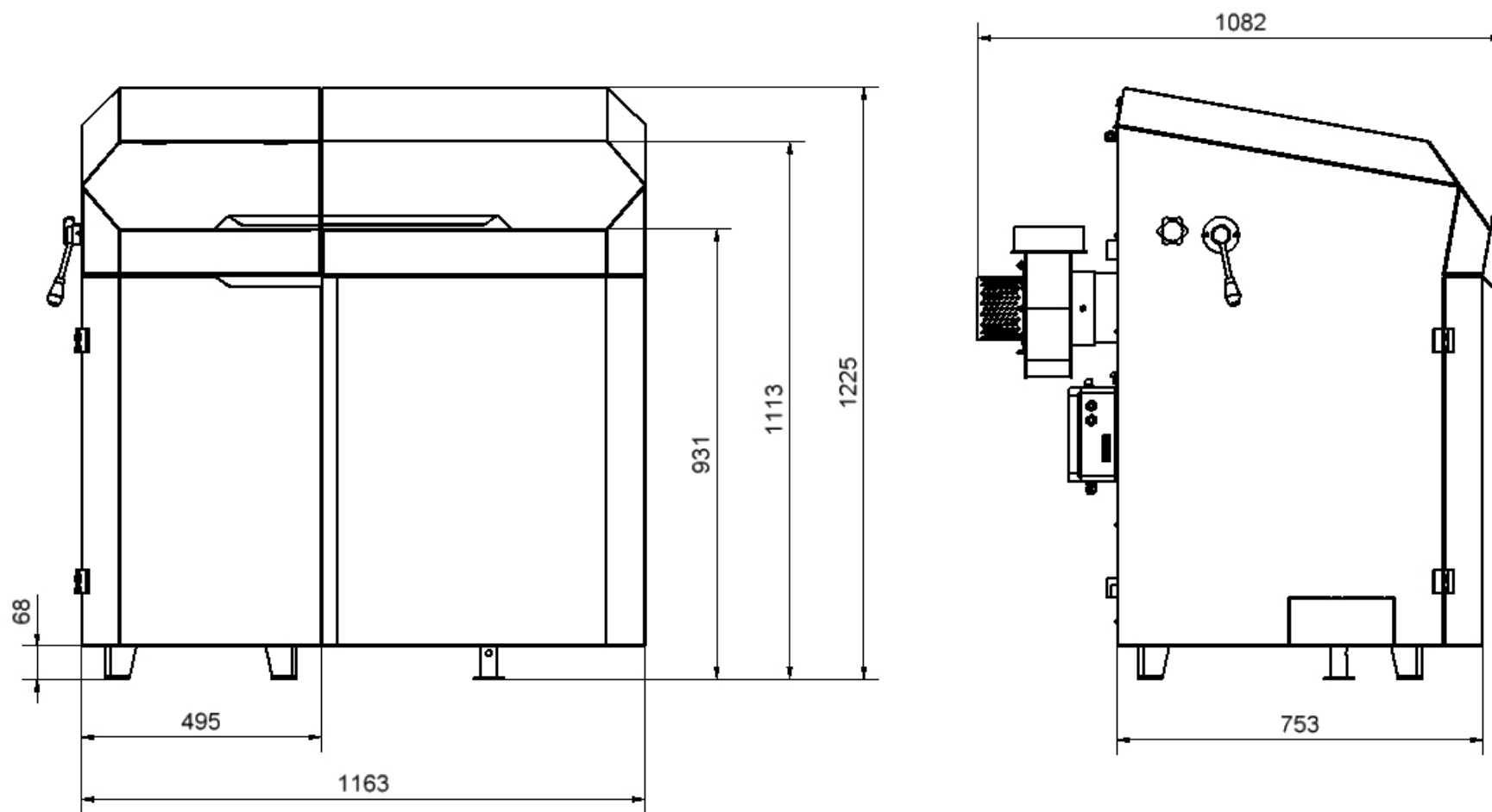
Obr. č. 3 Základní rozměry kotle CosmoTHERM G15
