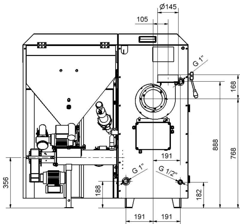
Obr. č. 6 Připojovací rozměry kotle CosmoTHERM G15
