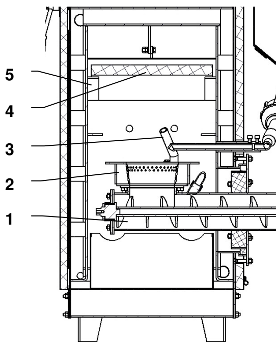
Obr. č. 8 Řez spalovací komorou kotle
