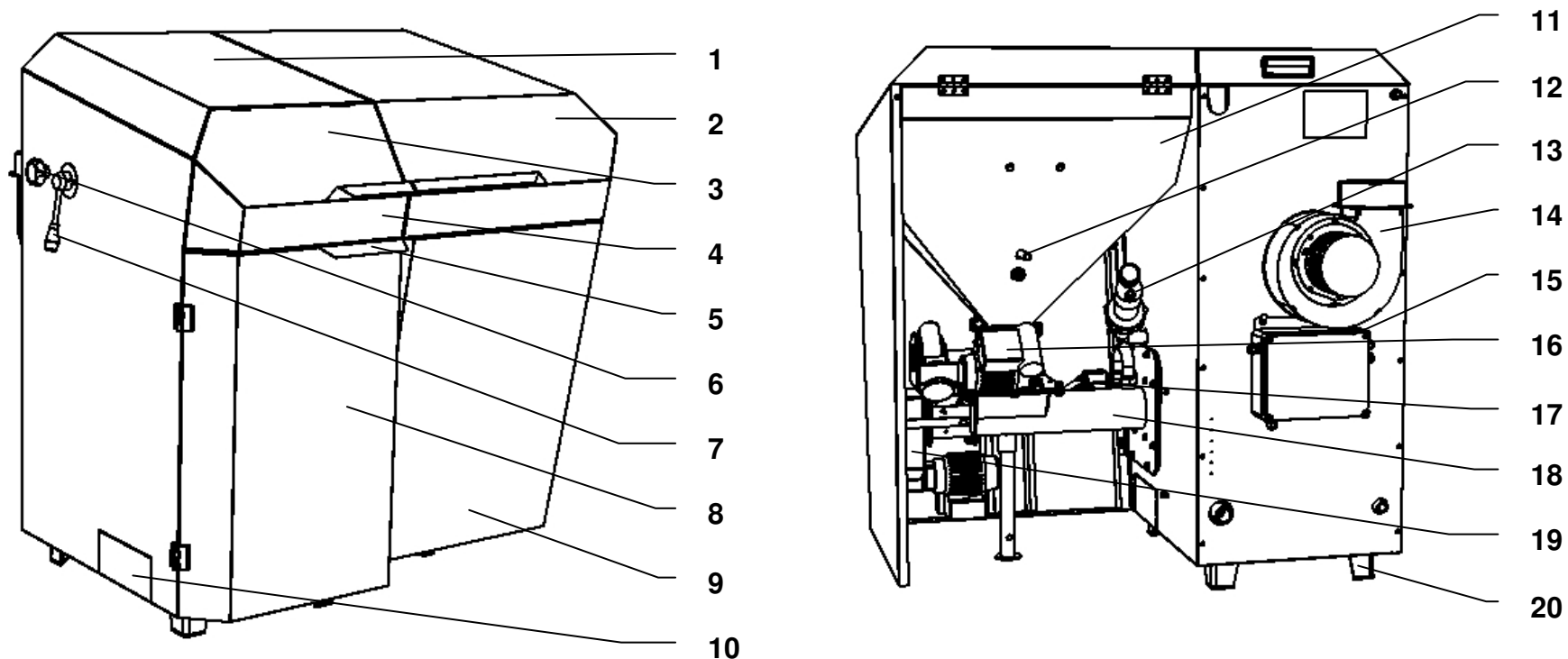
Obr. č. 1 Čelní a zadní pohled kotle CosmoTHERM G15
